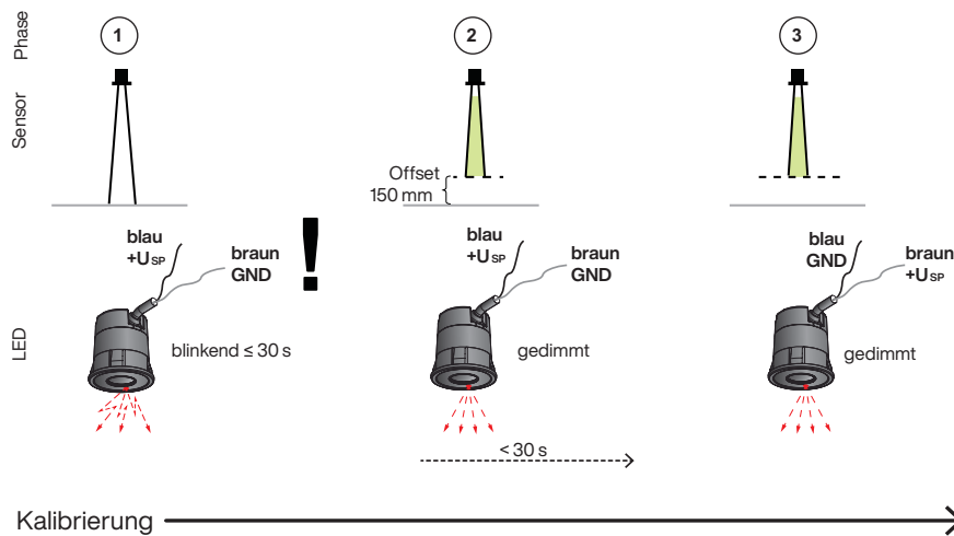
Abb 10: Konfiguration Typ T - Spannungswechsel
