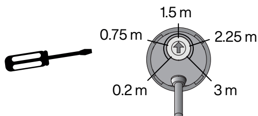
Abb 8: Beispiel für eine Einstellung zwischen 0.2 und 3 m
