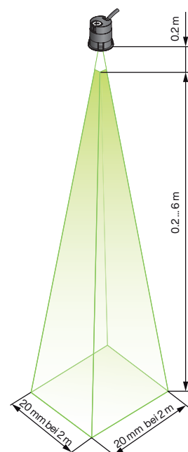
Abb 6: Abmessungen des Erfassungsbereichs
