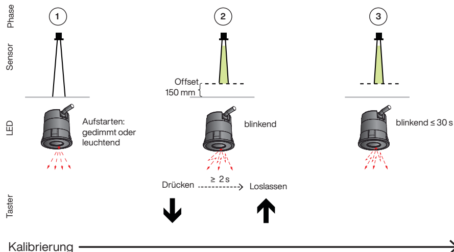
Abb 11: Konfiguration Typ T mit dem Teach-in-Taster
