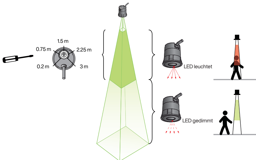
Abb 9: Konfiguration - Typ N
