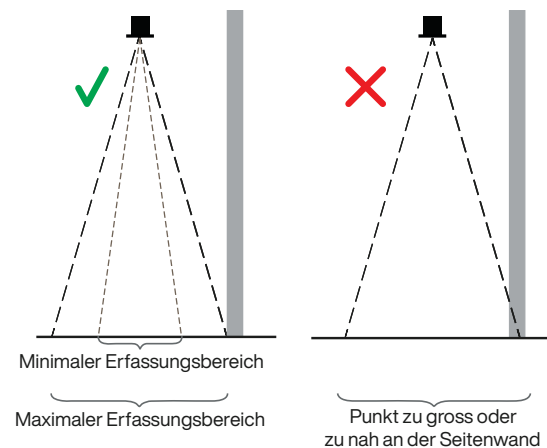
Abb 7: Beleuchtungsgröße des ToF-1S
