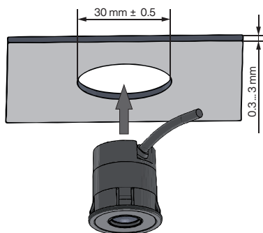
Abb 13: Montage des Snap-in Gehäuse
